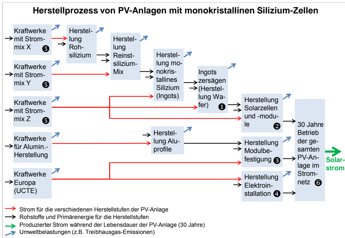
Abbildung 1: Die Umweltbelastung von Solarstrom hängt insbesondere von den Herstellstufen ① bis ⑥ ab.
